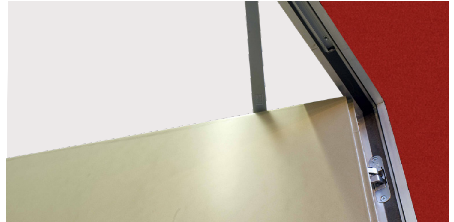
Porta tagliafuoco raso muro, lato corridoio, laccata con inserto personalizzato in metallo, certificata EI 30' - 31dB / Fire rated wall-flush door, corridor side lacquered with custom metallic insert, certified EI 30' - 31dB
